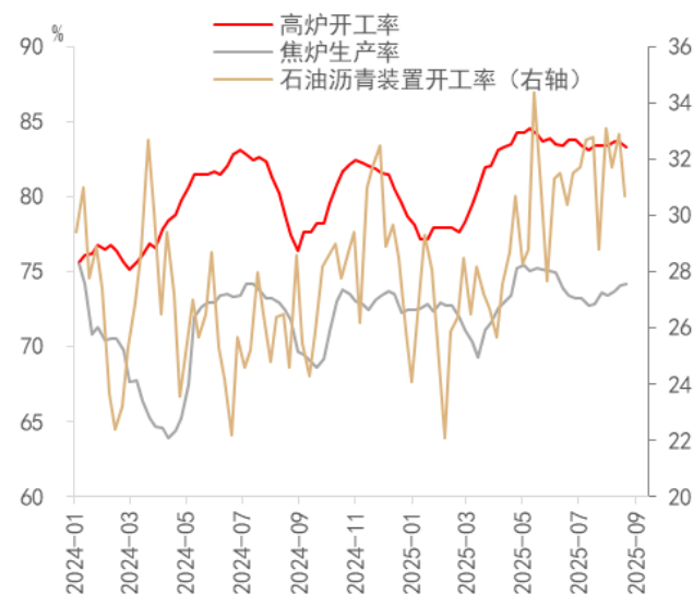
图表1：焦炉开工率升高，高炉、沥青下降
